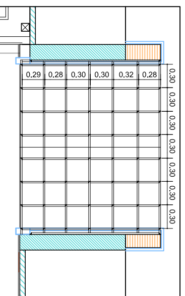
ΟΡΙΖΟΝΤΙΑ ΤΟΜΗ ΣΙΔΗΡΟΥ ΠΛΕΓΜΑΤΟΣ
