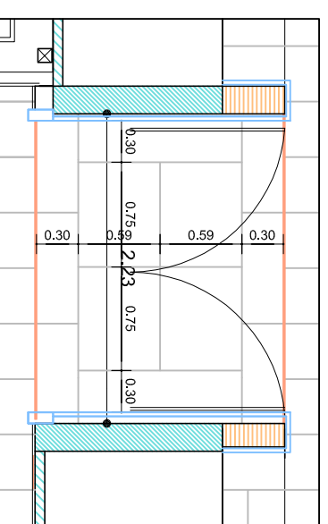
ΚΑΤΟΥΨΗ
