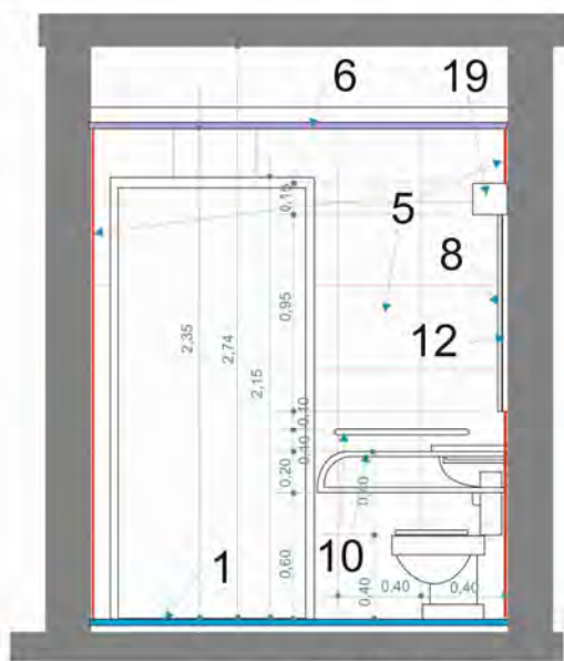
ΑΜΕΑ ΟΨΗ Γ
