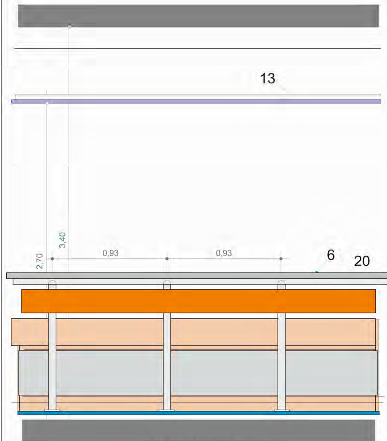
ΕΜΠΡΟΣΘΙΑ ΟΨΗ
