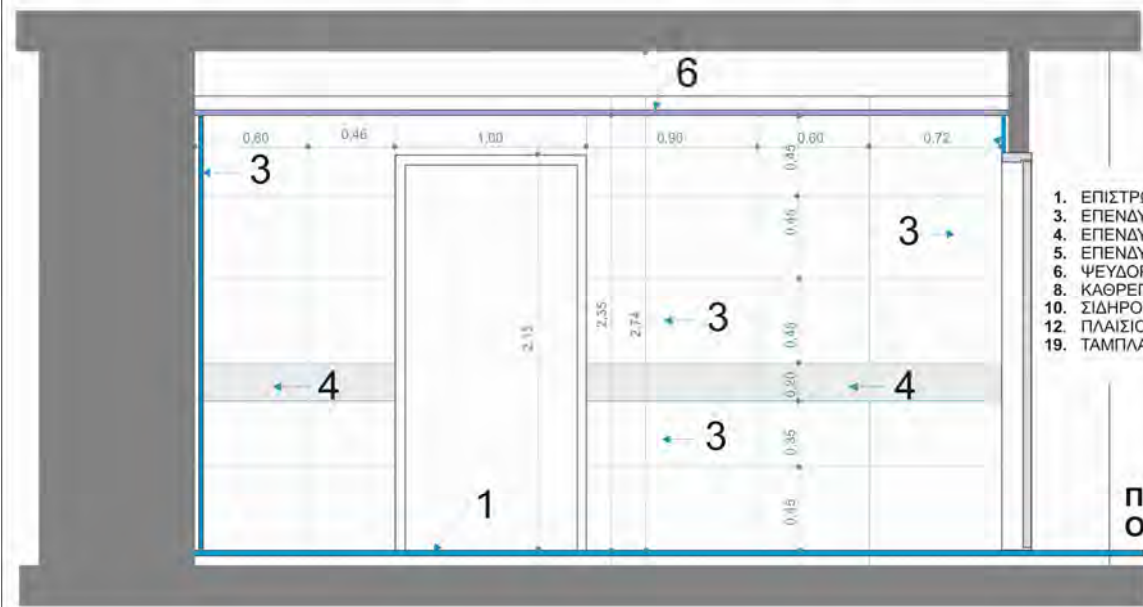
ΑΜΕΑ ΟΨΗ Δ
