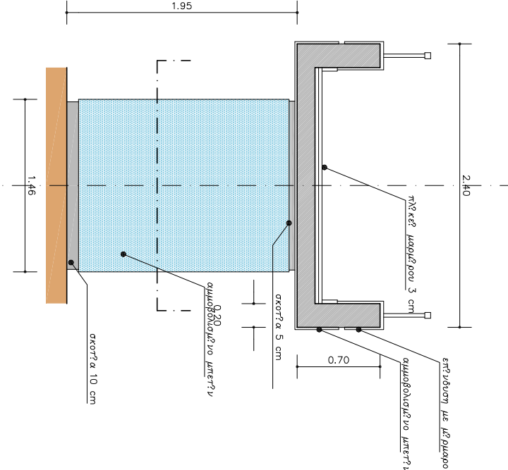
ΤΟΜΗ Β-Β
