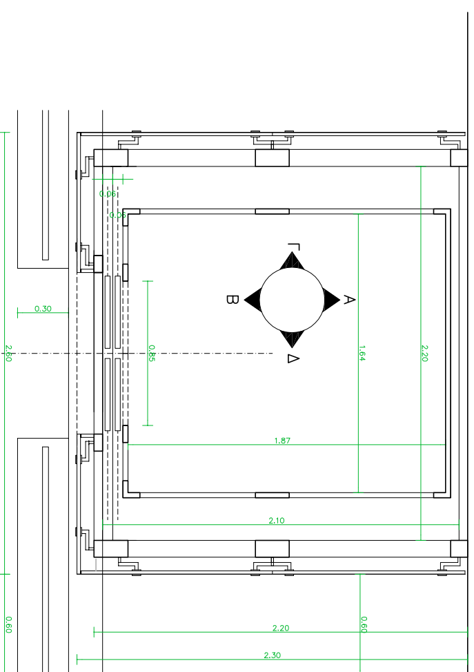
ΚΑΤΟΥΗ ΦΡΕΑΤΟΣ ΚΑΙ ΚΑΜΠΙΝΑΣ
