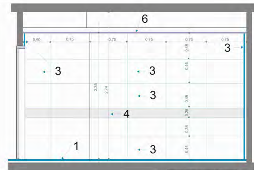
ΠΡΟΘΑΛΑΜΟΣ ΟΨΗ Β
